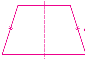
trapesium samakaki
