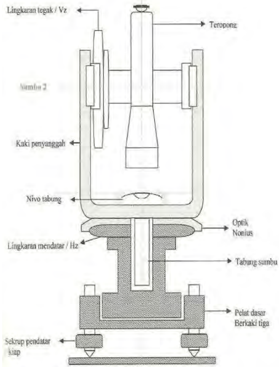
Gambar 3.1. Konstruksi Teodolit
