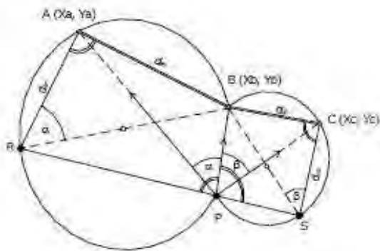
Gambar 3.4. Cara Cassini
