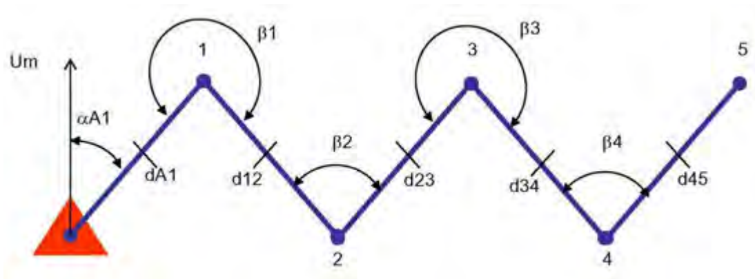
Gambar 3.10. Poligon terbuka terikat sempurna
