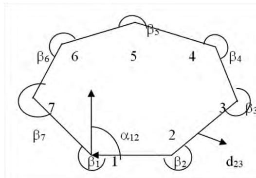
Gambar 3.8. Poligon tertutup
