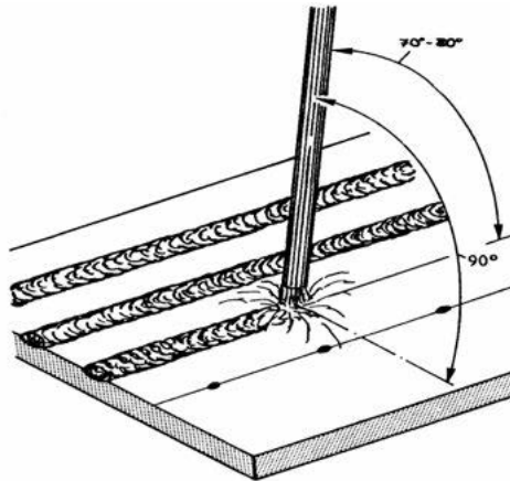
Gambar Posisi elektroda terhadap benda kerja
